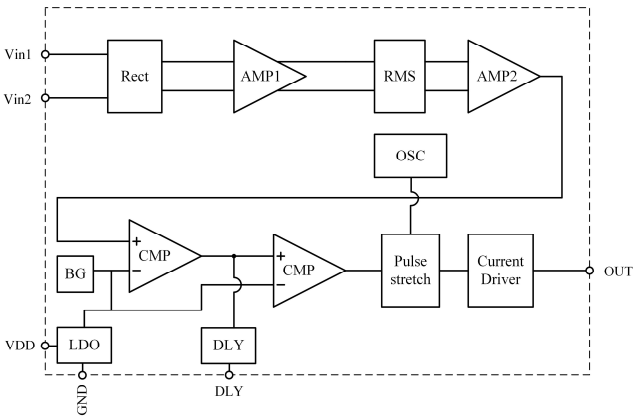
功能框图
