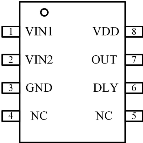
图 1 引脚配置（顶视图）
