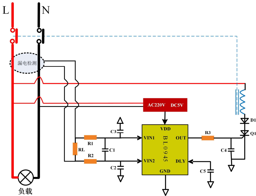
图 2 典型应用示意图
