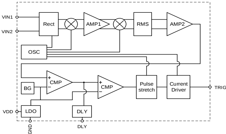
功能框图
