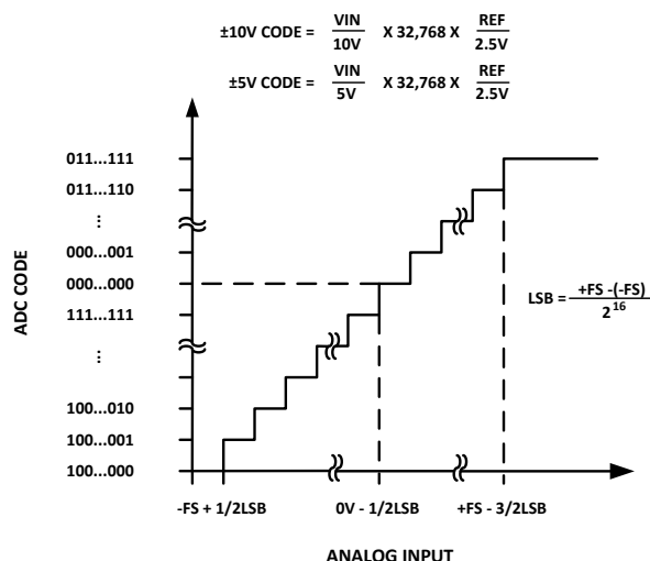
图 32. BL1086 传递特性
