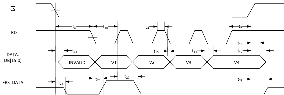
图 4. 并行模式，独立 \overline{CS} 和 \overline{RD} 脉冲
