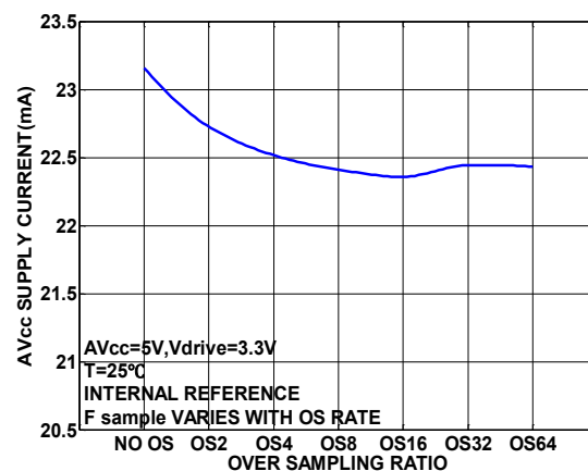
图 26. 电源电流与过采样倍率的关系
