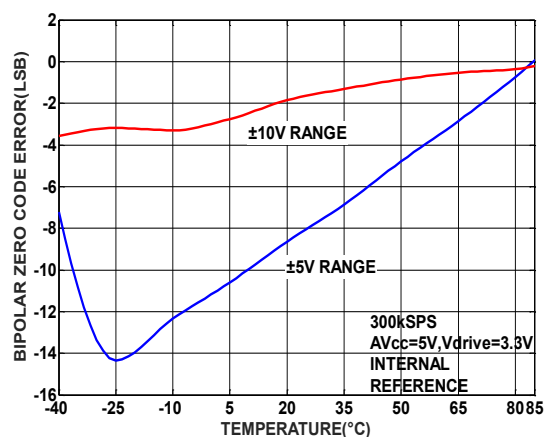
图 17. 双极性零代码误差与温度的关系
