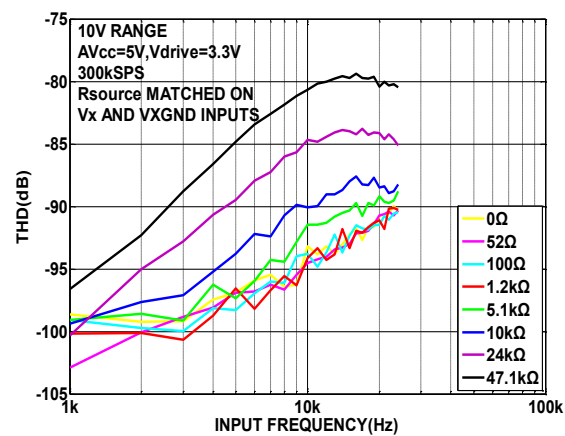
图 19. 各种源阻抗下 THD 与输入频率的关系, \pm 10V 范围
