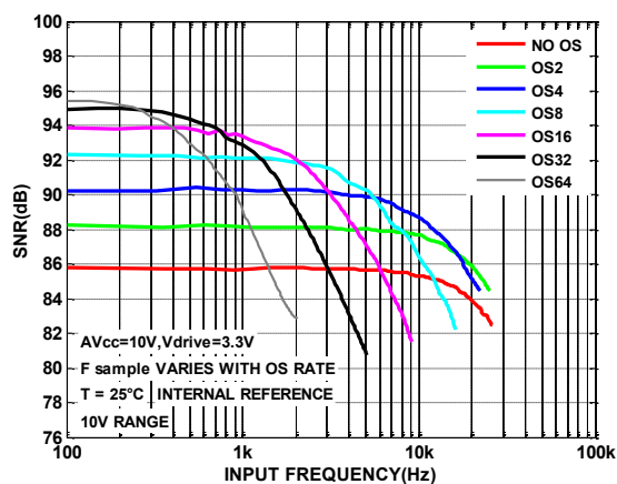
图 22. 不同过采样倍率下 SNR 与输入频率的关系, \pm 10V 范围
