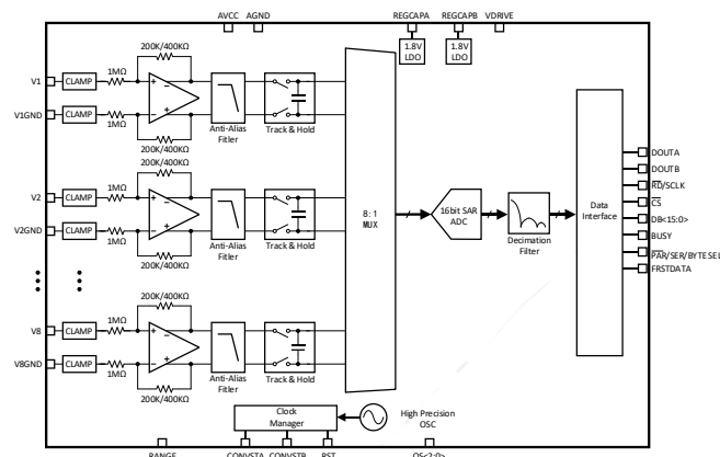
图 1. 功能框图
