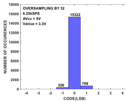
图 47. 码直方图：32 倍过采样
