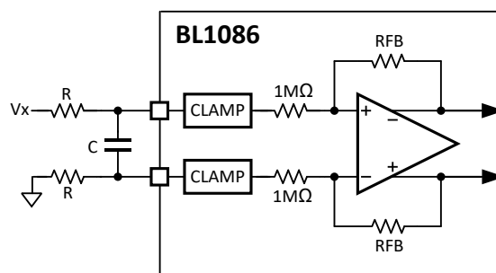
图 30. BL1086 模拟输入端上的输入电阻匹配
