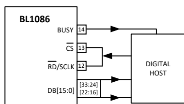
图 38. 一个 BL1086 使用并行总线 \overline{\text{RD}} 和 \overline{\text{CS}} 短接在一起
