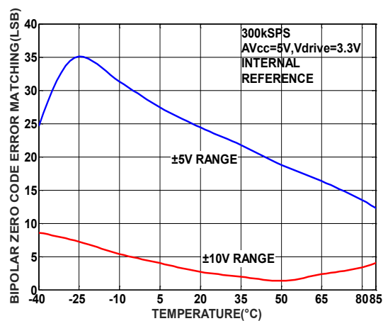
图 18. 通道间的双极性零代码误差匹配
