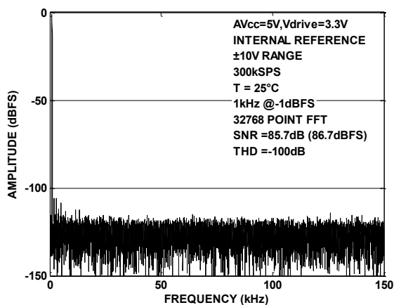
图 9. BL1086 FFT \pm 10V 范围
