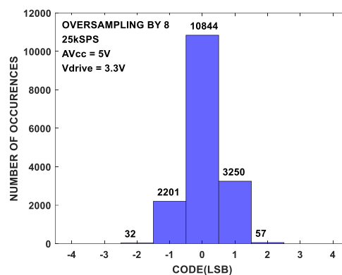
图 45. 码直方图：8 倍过采样
