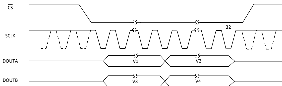
图 39. 采用双 DOUT 线路的 BL1086 串行接口
