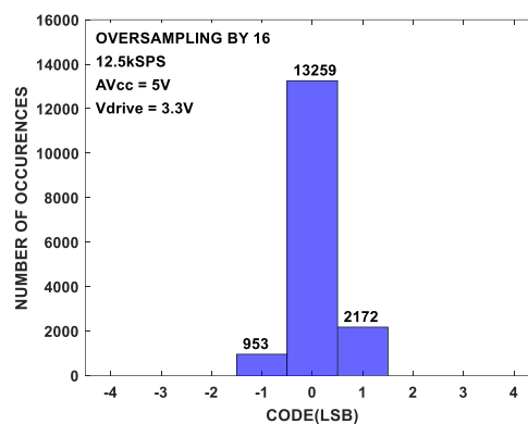
图 46. 码直方图：16 倍过采样
