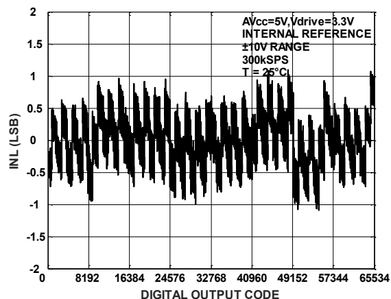
图 12. BL1086 典型 INL, \pm 10V 范围
