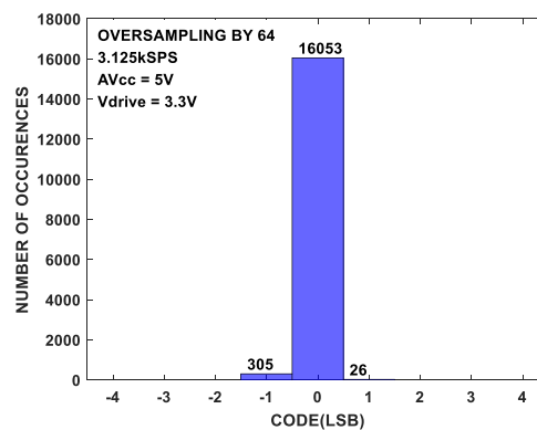
图 48. 码直方图：64 倍过采样
