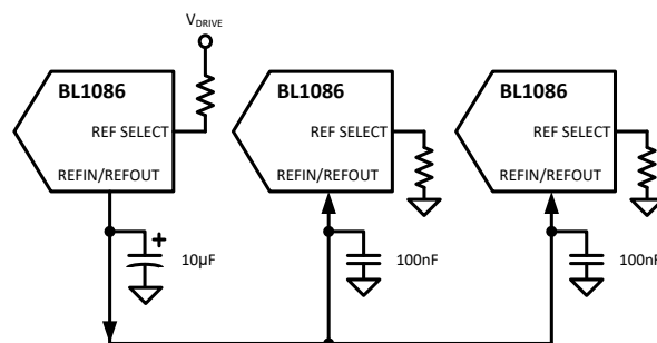
图 35. 内部基准电压源驱动多个 BL1086 REFIN 引脚
