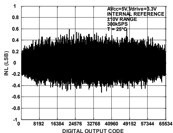
图 13. BL1086 典型 DNL, \pm 10V 范围
