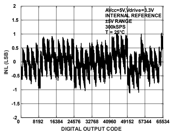
图 14. BL1086 典型 INL, \pm 5V 范围
