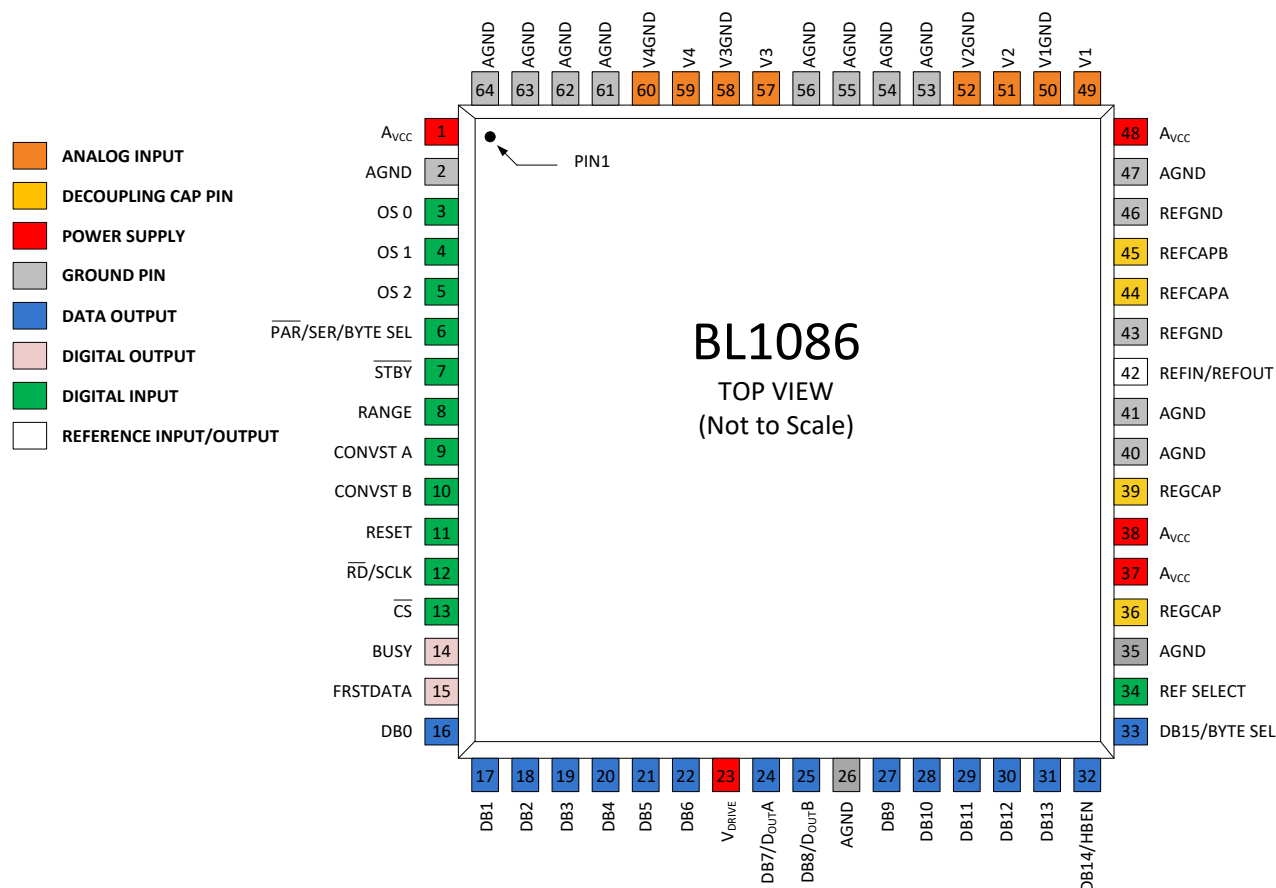
图 8. BL1086 引脚配置 (顶视图)
