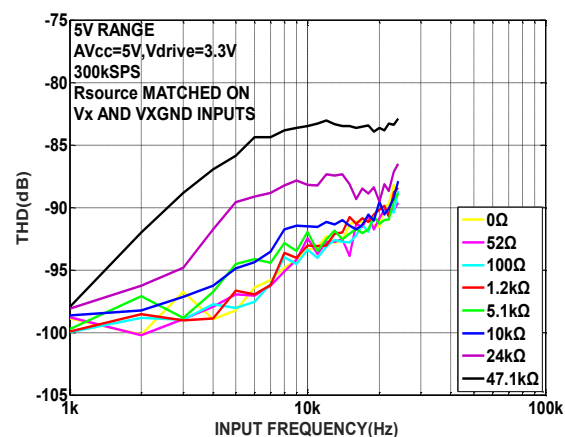
图 20. 各种源阻抗下 THD 与输入频率的关系, \pm 5V 范围
