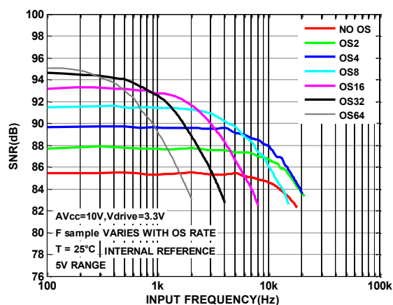
图 21. 不同过采样倍率下 SNR 与输入频率的关系, \pm 5V 范围
