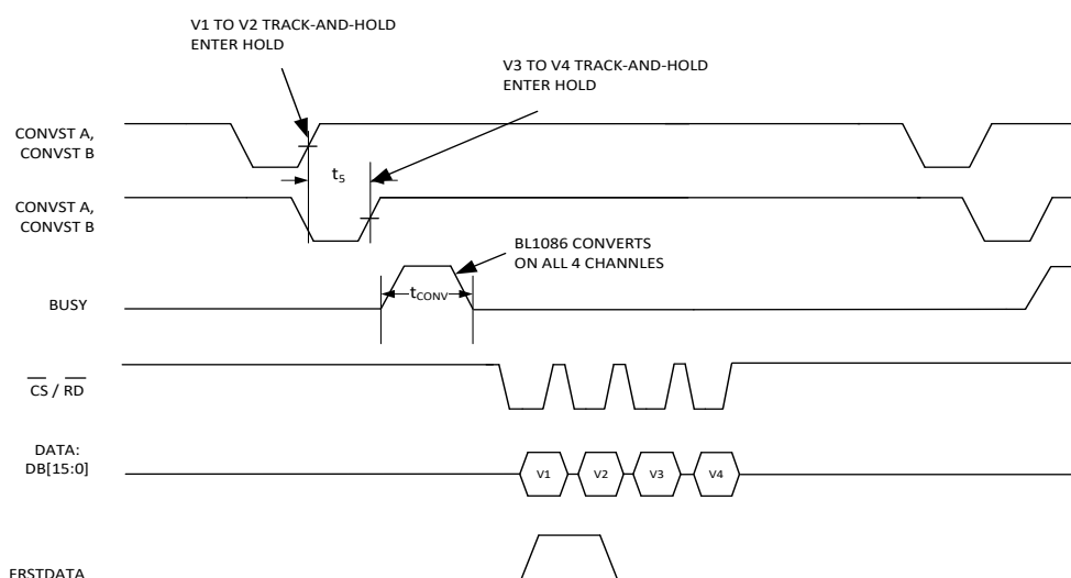
图 37.BL1086 分两组通道同步采样, 使用独立的 CONVSTA 和 CONVSTB-并行模式
