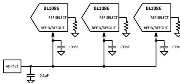
图 34. 一个外部基准电压源驱动多个 BL1086 REFIN 引脚
