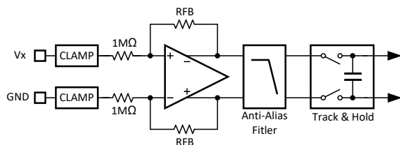
图 28. 模拟输入电路
