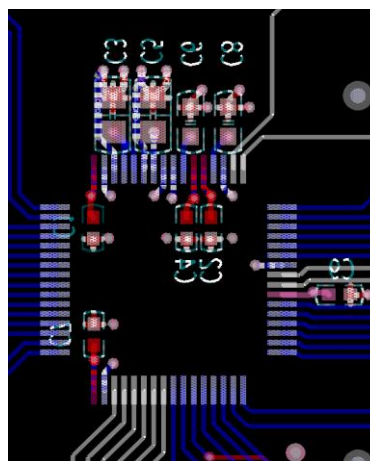
图 49. BL1086 外围去耦
