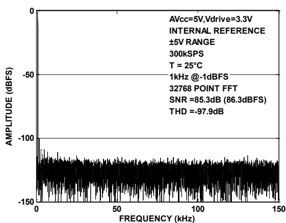
图 10. BL1086 FFT \pm 5V 范围
