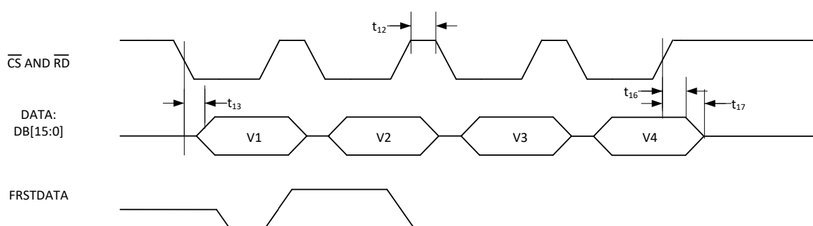
图 5. \overline{CS} 和 \overline{RD} 相连的并行模式
