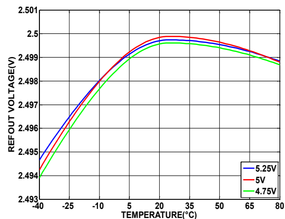
图 24. 不同电源电压下基准输出电压与温度的关系
