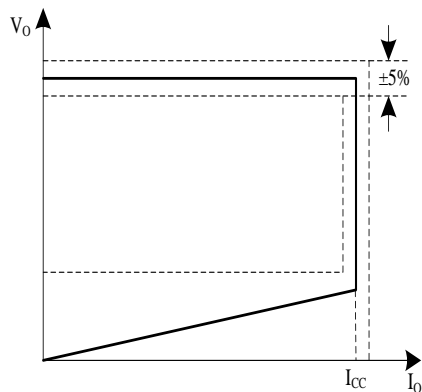
cc/cv 曲线
