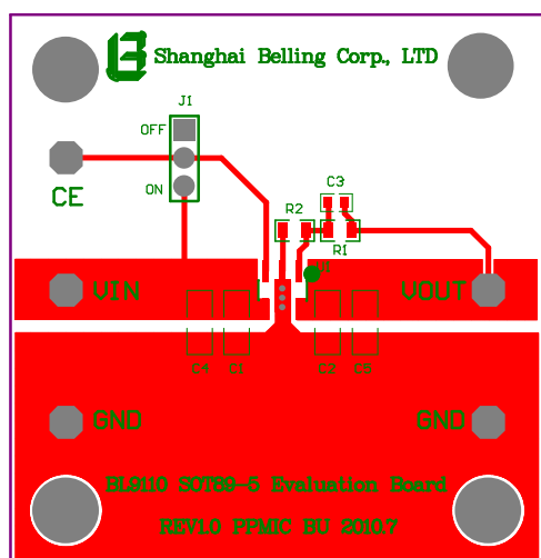
Top Layer
