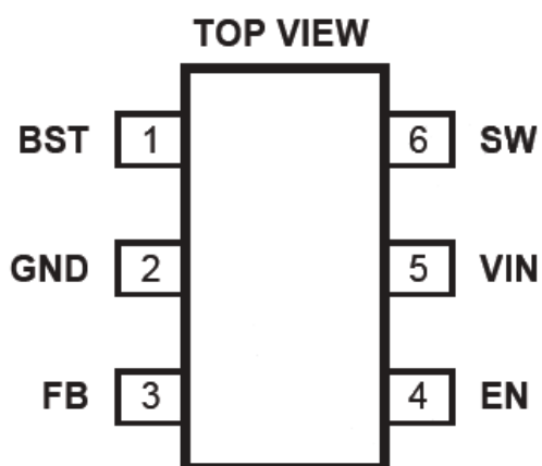
外形图和丝印说明
