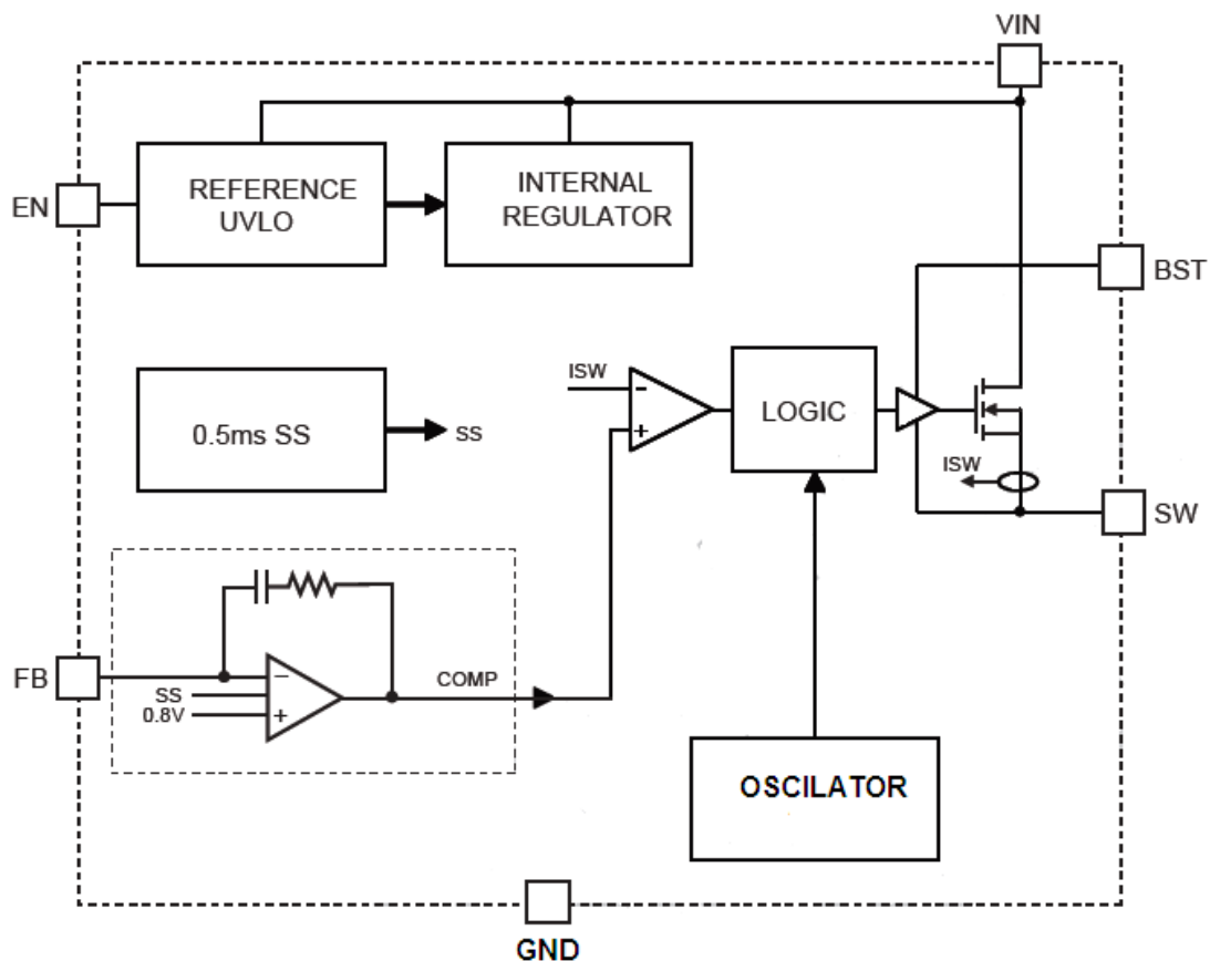
框图
