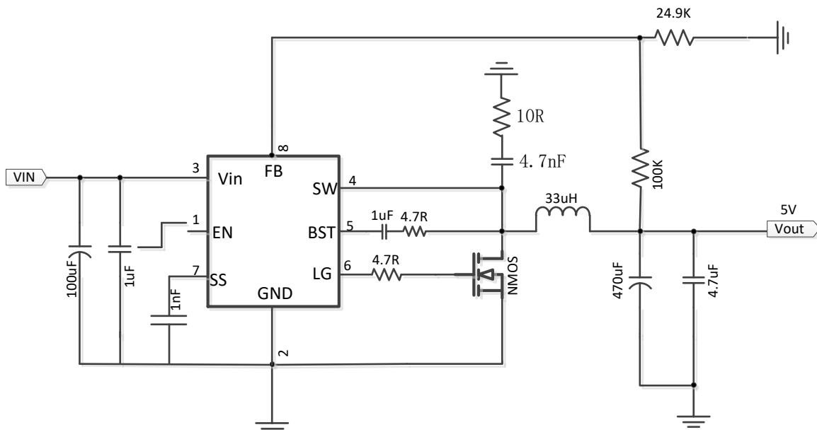
Figure3. 12V-70V VIN, 5V/2A
