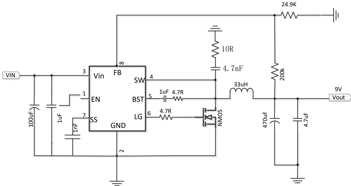
Figure4. 12V-70V VIN, 9V/2A
