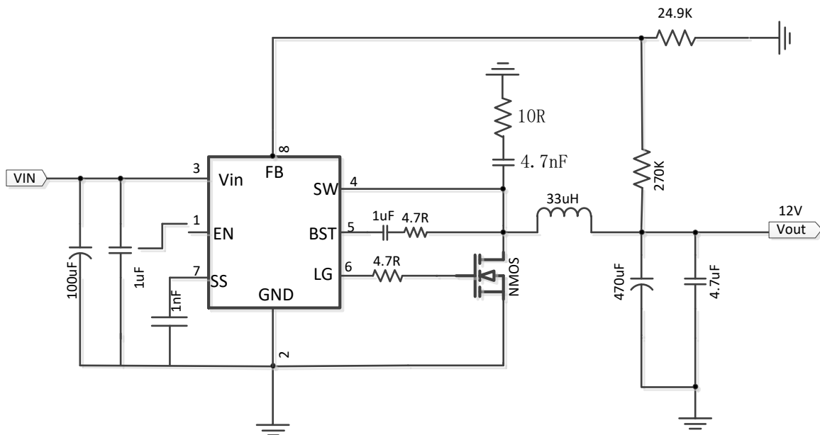
Figure5. 14V-70V VIN, 12V/2A
