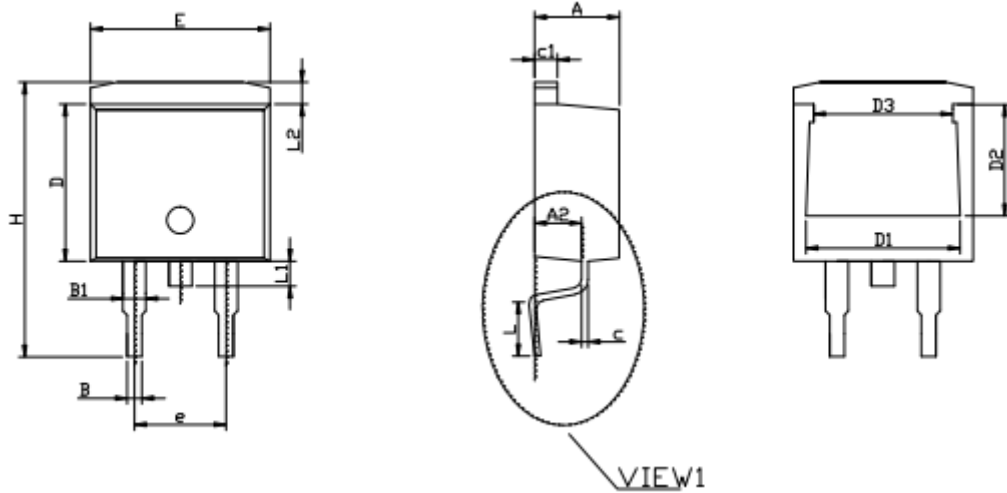
TO-263
