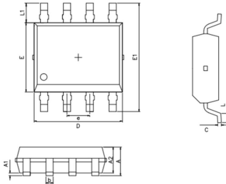
SOP 8
